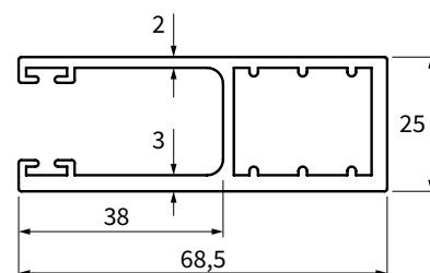
doorsnede HTF 68 Zwaar geleider (G)
